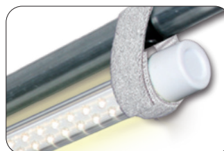
Kit fissaggio con nastro a strappo Fastening kit with tear-away tape
