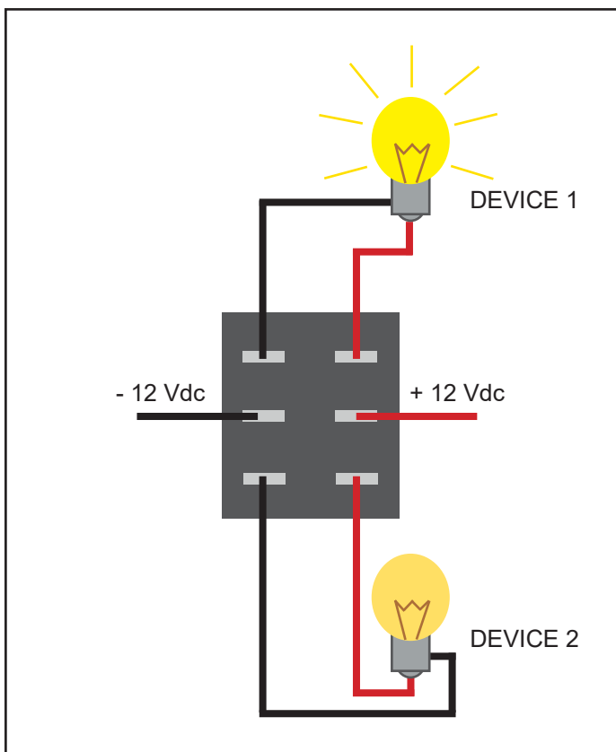
COLLEGAMENTO TRADIZIONALE TRADITIONAL CONNECTION
