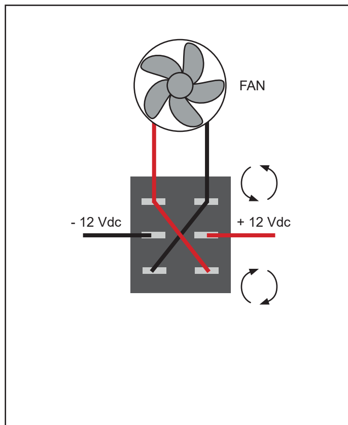
COLLEGAMENTO CON INVERSIONE DI POLARITÀ CONNECTION WITH POLARITY INVERSION
